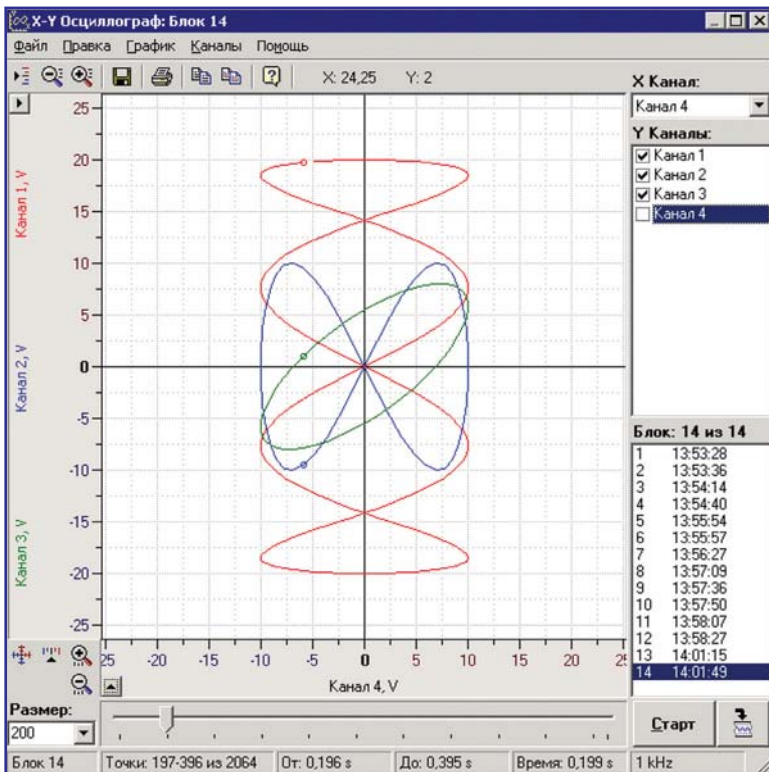
"X-Y Осциллограф" позволяет строить и регистрировать параметрические графики зависимости одного сигнала от другого.
