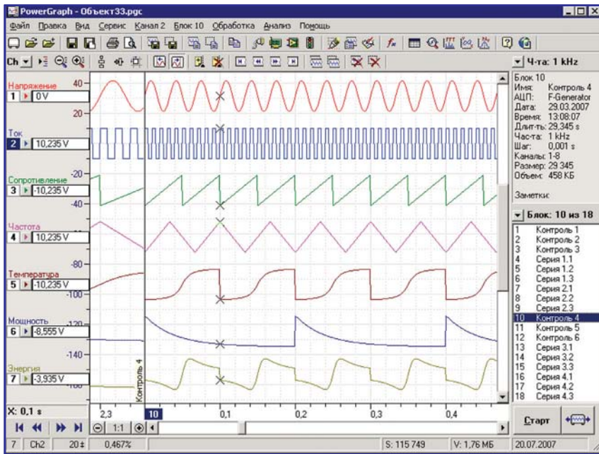
Главное окно программы содержит все необходимые элементы управления, графики каналов, список и параметры записанных блоков данных.
